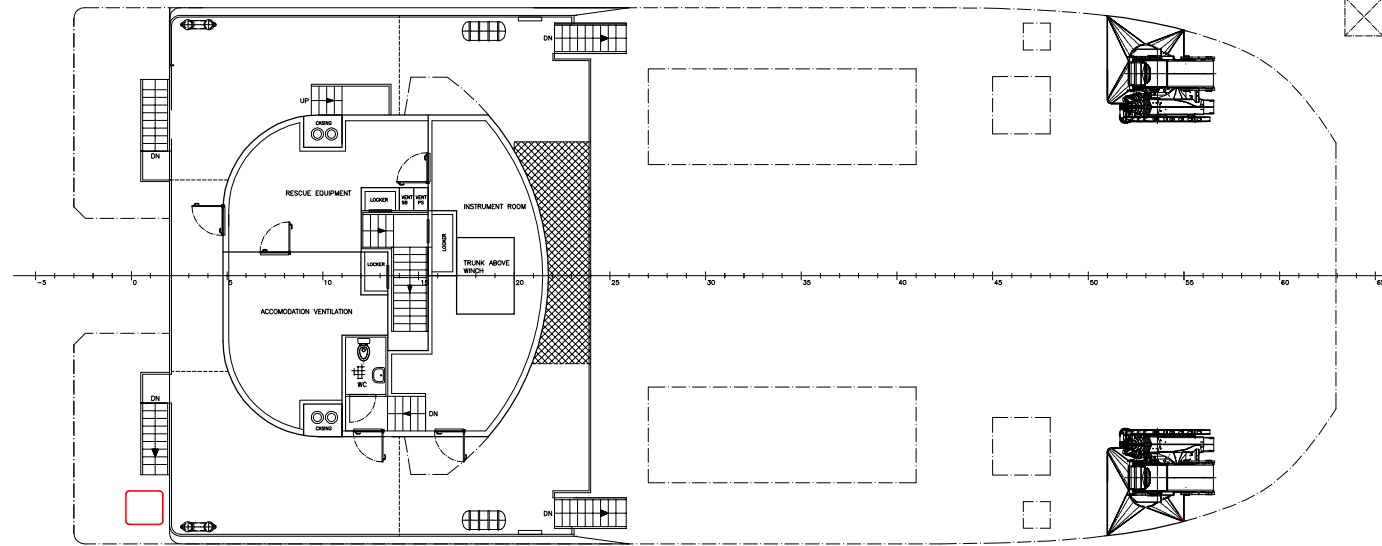
A-DECK
