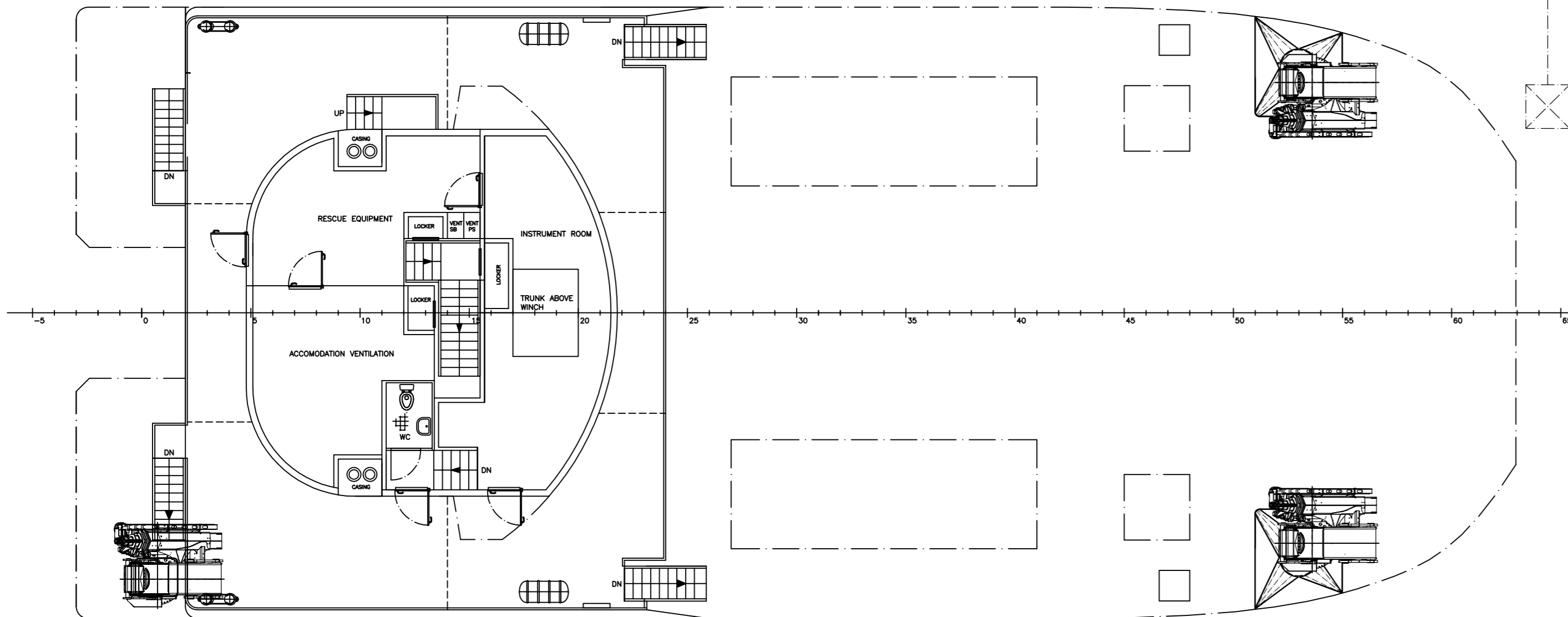
A-DECK
